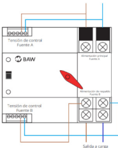
Figura 2 - Esquema de conexión
