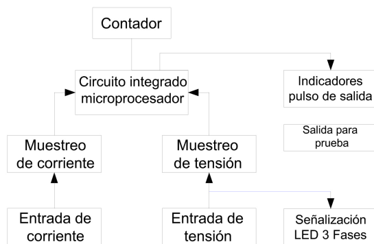
Diagrama de principio de funcionamiento
